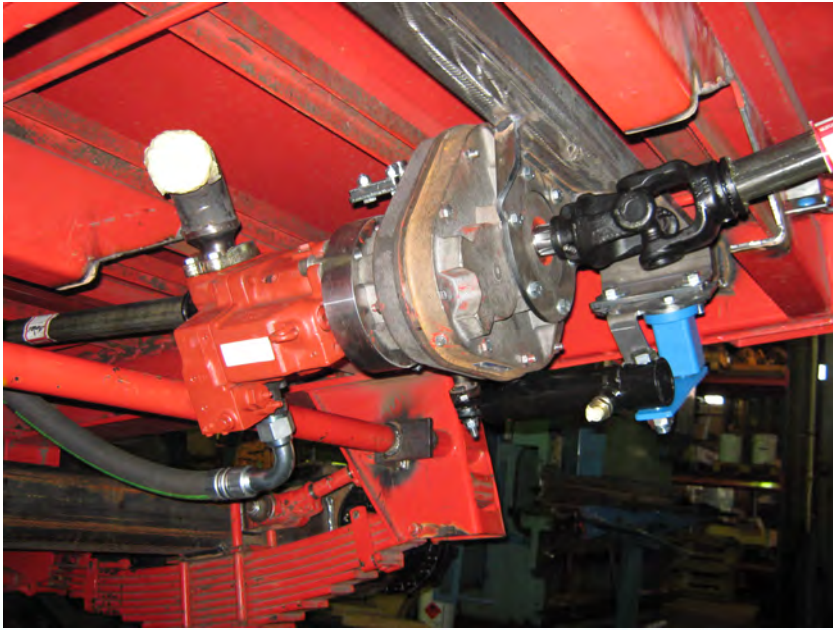
Vaihteiston ja pumpun asennusta kärryn voimansiirtolinjaan
